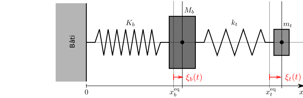
FIGURE 4 – Haut : schéma de principe du détecteur Explorer (source : adapté du site http://www.lnf.infn.it/esperimenti/rog ). Bas : modélisation de la barre d'aluminium muni du transducteur par deux oscillateurs mécaniques de masses M_b et m_t couplés par des ressorts de raideur K_b et k_t , avec M_b \gg m_t . Les deux oscillateurs sont accordés sur la même fréquence de résonance. Les positions d'équilibre des masses M_b et m_t sont respectivement x_b^{eq} et x_t^{eq} .
